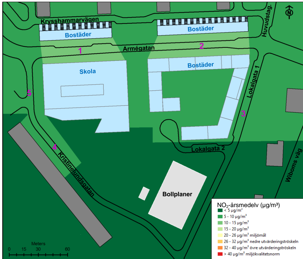
Figur 11. Årsmedelvärden NO 2 i µg/m 3 i utbyggnadsalternativet år 2040. Normvärdet som skall klaras är 40 µg/m 3 och miljömålet 20 µg/m 3 .
