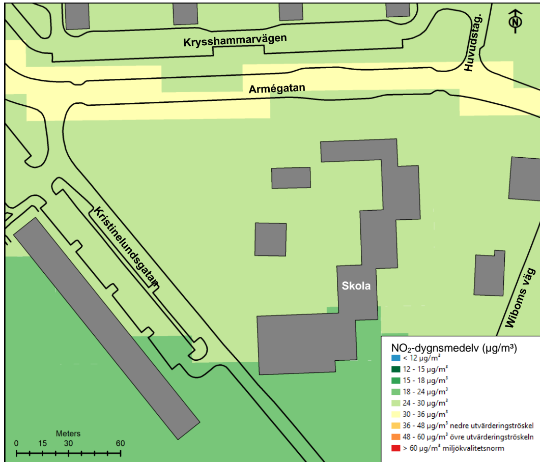
Figur 6. Dygnsmedelvärden NO 2 i µg/m 3 det 8:e högsta dygnet i nuläget år 2020. Normvärdet som skall klaras är 60 µg/m 3 .
