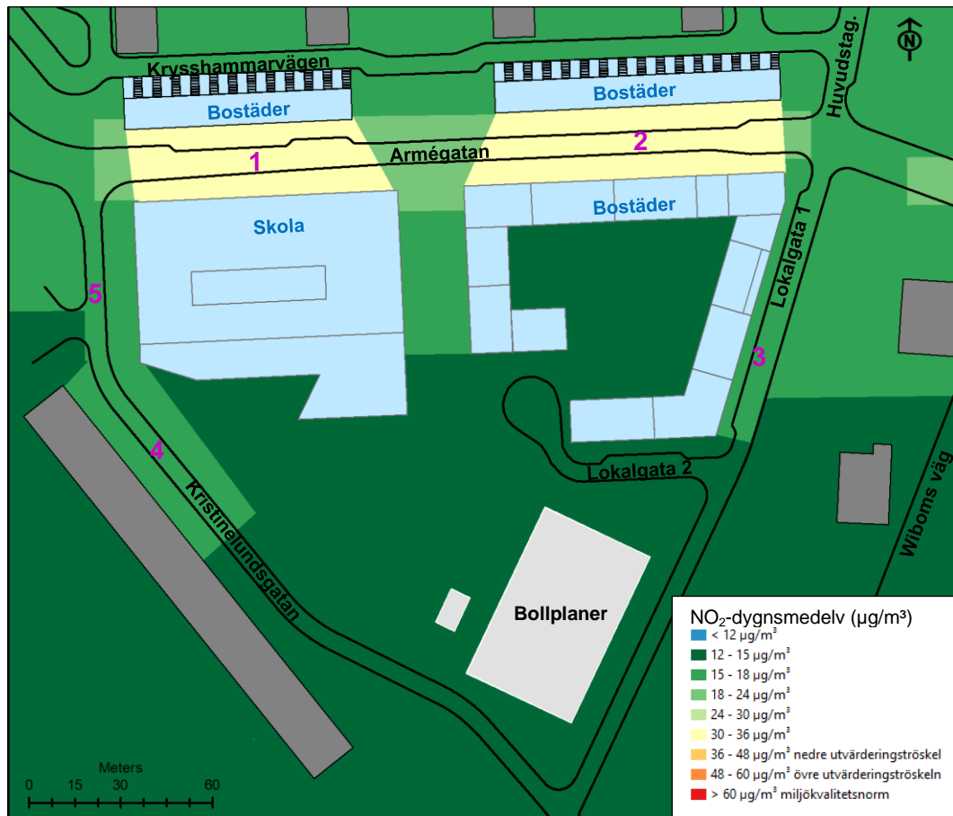
Figur 12. Dygnsmedelvärden NO 2 i µg/m 3 det 8:e högsta dygnet i utbyggnadsalternativet år 2040. Normvärdet som skall klaras är 60 µg/m 3 .
