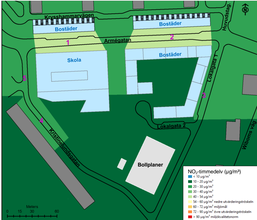
Figur 13. Timmedelvärderna NO 2 i µg/m 3 den 176:e högsta timmen i utbyggnadsalternativet år 2040. Normvärdet som skall klaras är 90 µg/m 3 och miljömålet 60 µg/m 3 .
