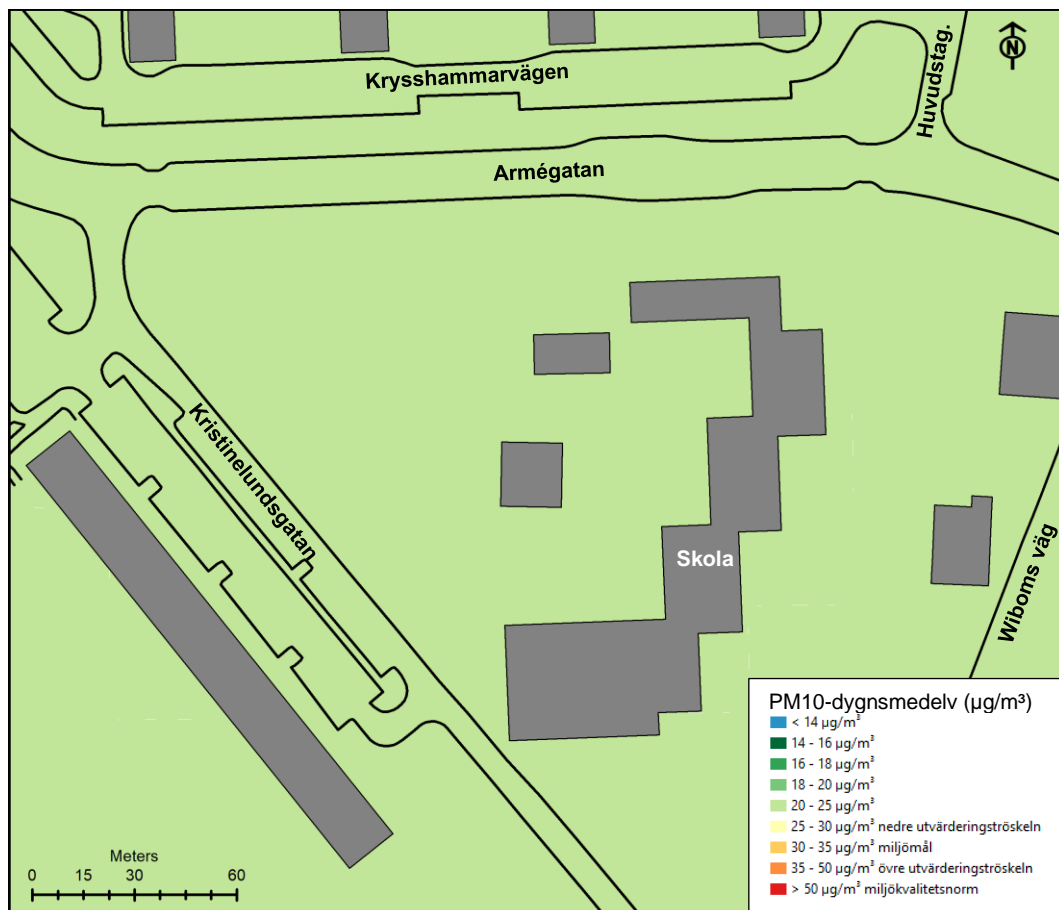
Figur 5. Dygnsmedelvärden PM10 i µg/m 3 för det 36:e högsta dygnet i nuläget år 2020. Normvärdet som skall klaras är 50 µg/m 3 och miljömålet 30 µg/m 3 .
