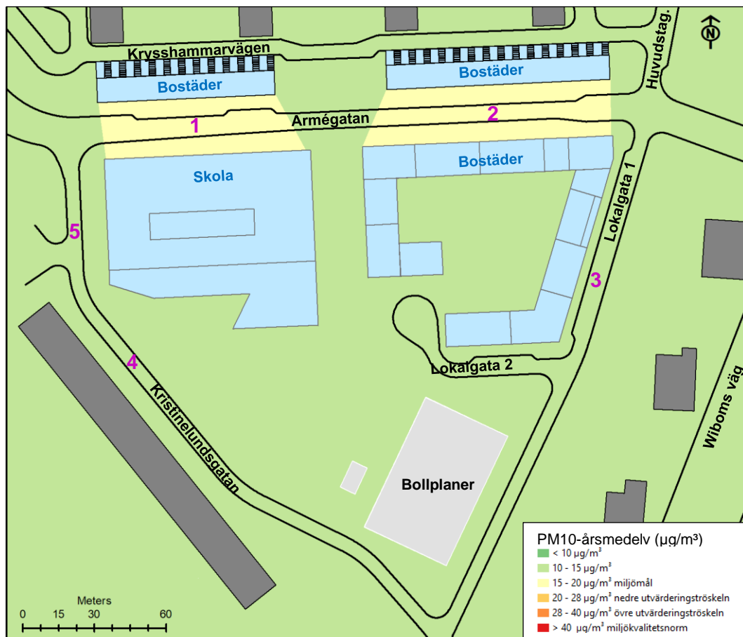
Figur 9. Årsmedelvärden PM10 i \mu\text{g}/\text{m}^3 i utbyggnadsalternativet år 2040.
