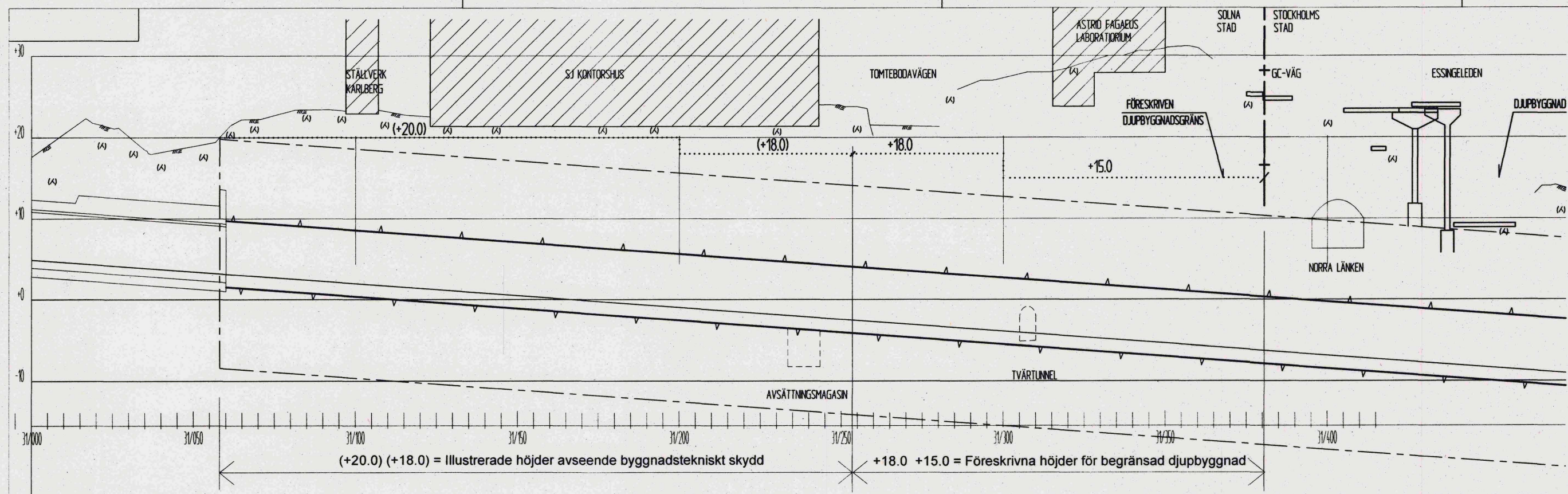
Sektion genom järnvägstunnel (spår U22) Skala H=1:400 L=1:1000
